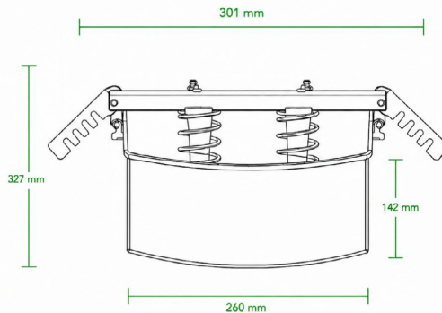
VISTA LATERAL
