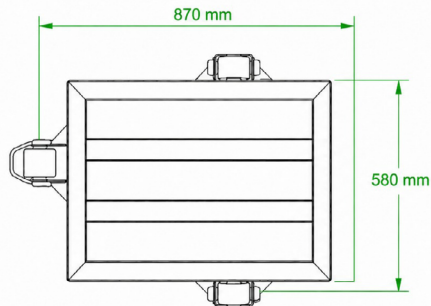
VISTA SUPERIOR
